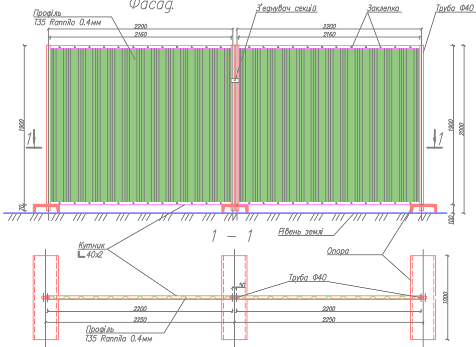
Огородження тимчасове глухе секційне на окремо розташованих опорах Фасад.
