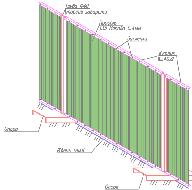
Огородження тимчасове глухе секційне, із профіля Rannila, на окремо розташованих опорах Підбір елементів.
