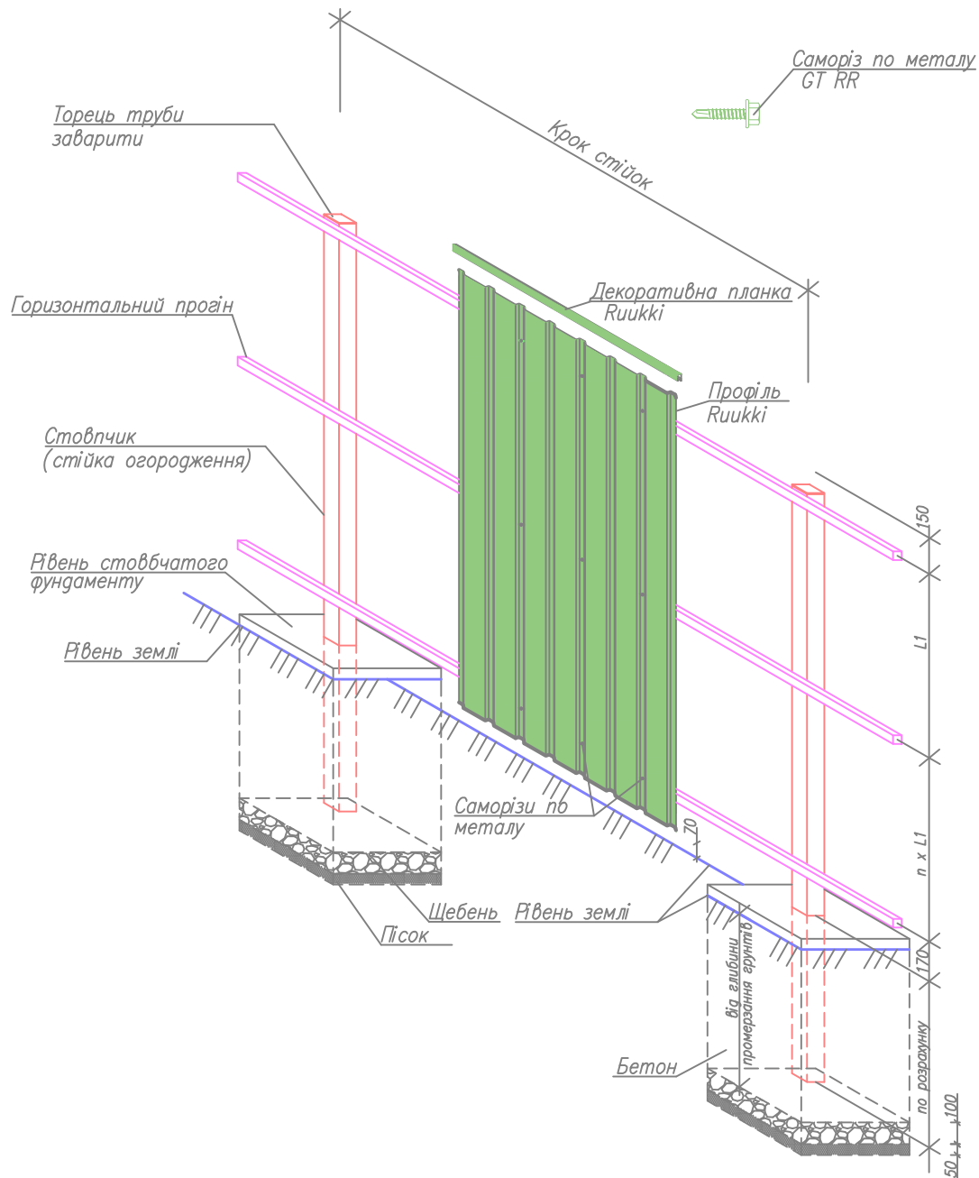
Огородження із профіля Ruikki на окремо розташованих фундаментах (варіант). Підбір елементів.
